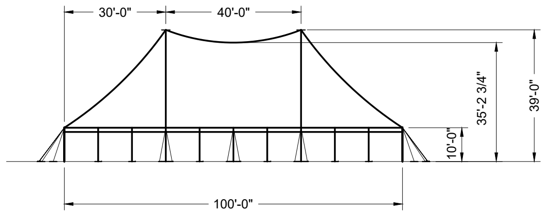
END ELEVATION
