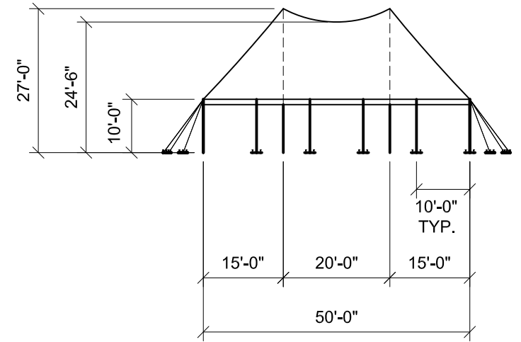
END ELEVATION
