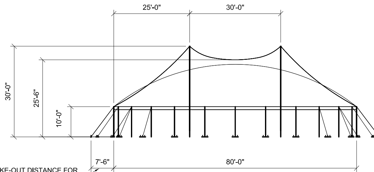
END ELEVATION
