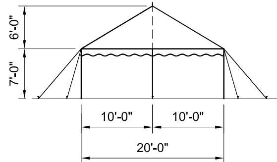
END ELEVATION
