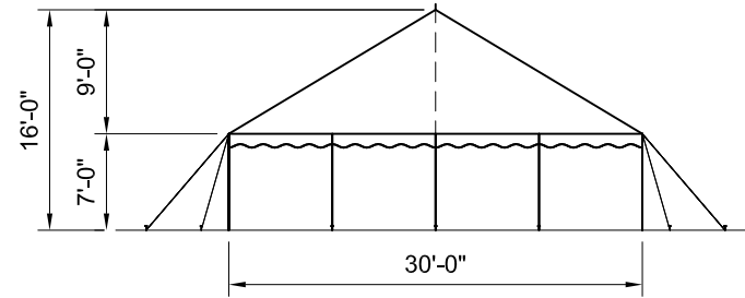
END ELEVATION
