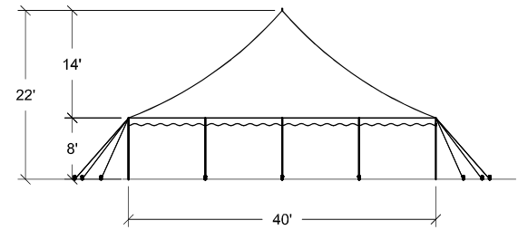
END ELEVATION
